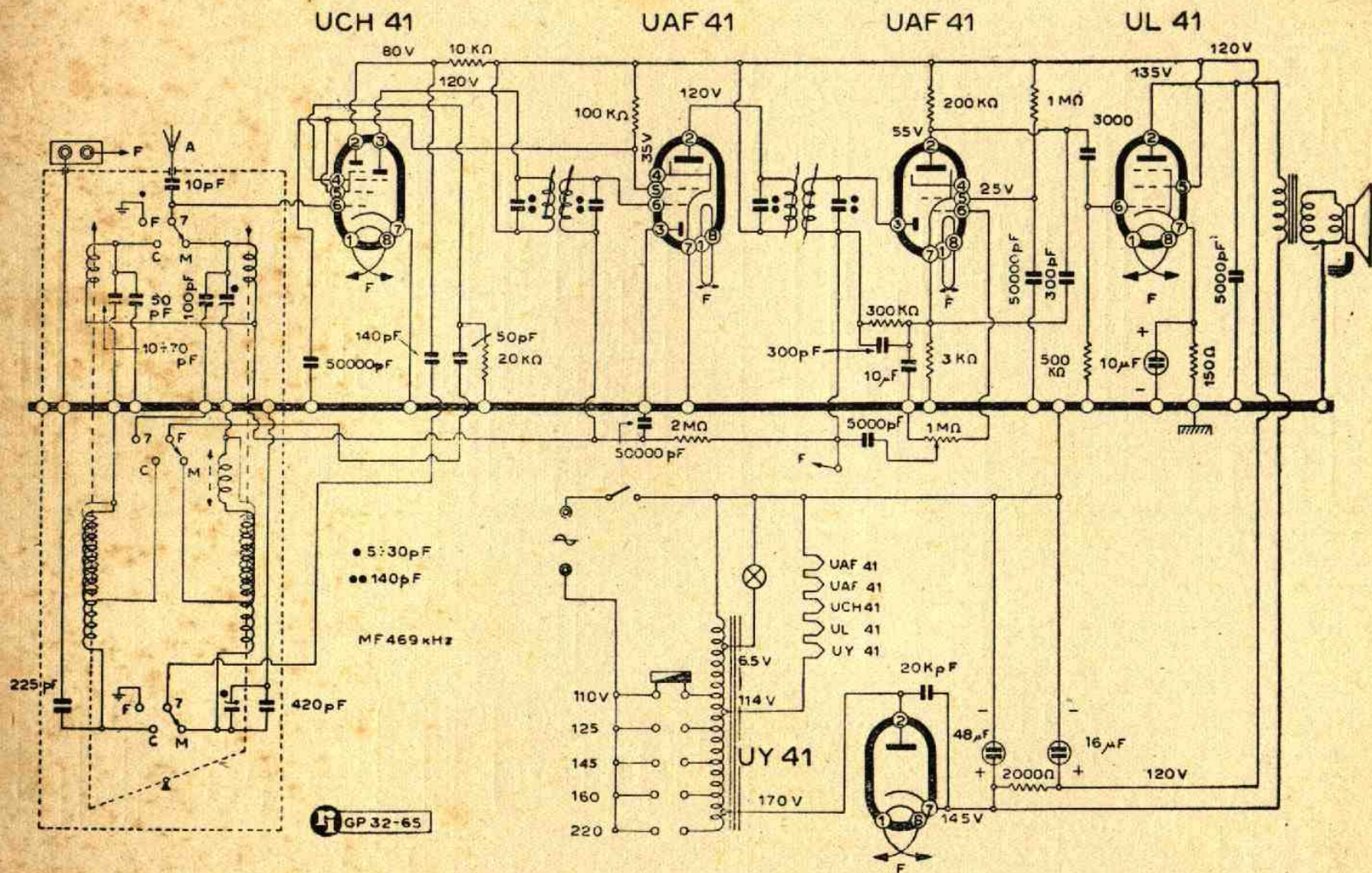
Lo schema elettrico del mod. S 529.
